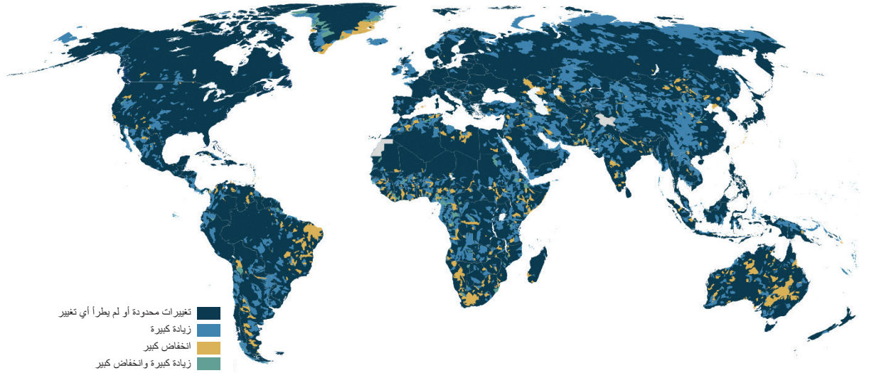
الشكل 1- التغيرات في المياه السطحية على الصعيد العالمي
